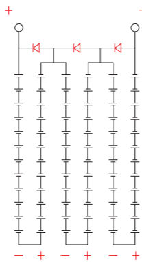
Diagrama de circuito
