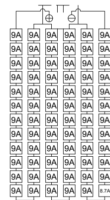
Diagrama de desajuste eléctrico
