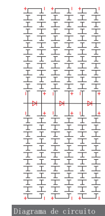
Diagrama de circuito
