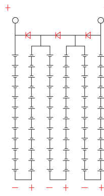
Diagrama de circuito
