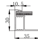
Long Frame A-A
